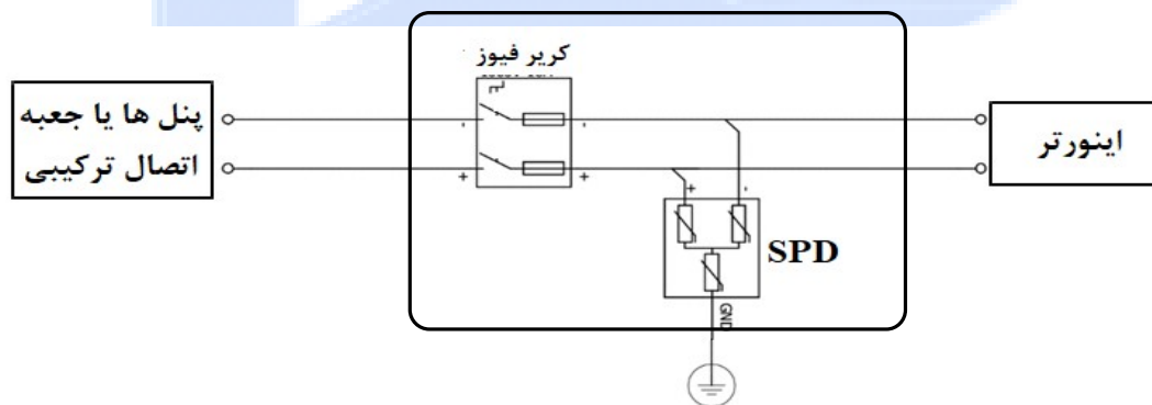
شکل (۴): شمای تک خطی یک تابلو DC
