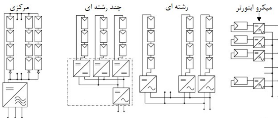
شکل (۱): انواع اینورترهای خورشیدی متصل به شبکه
