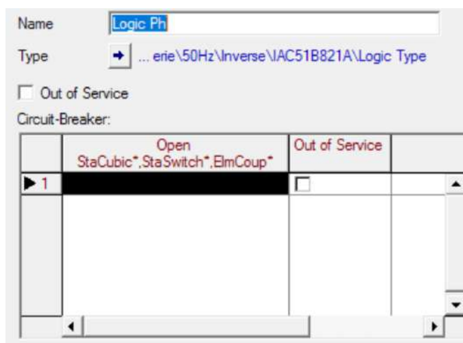
شکل (۷-۲۶): بخش المان ماژول منطق خطای فاز
