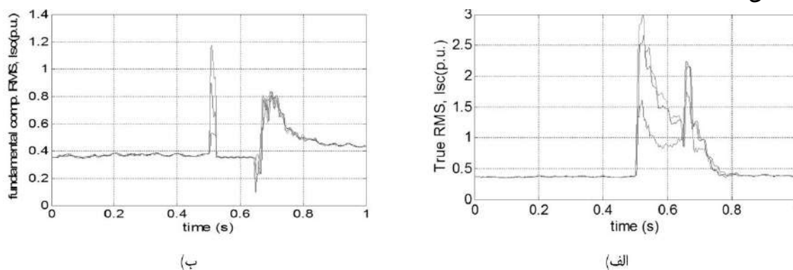
شکل (۴-۱۳): مقدار هارمونیک اصلی جریان اتصال کوتاه (۱) بدون کربار، (۲) با وجود کربار
