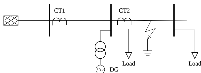
شکل (۴-۵): گذر جریان مختلف از دو ترانس جریان و احتمال اشباع و ناهماهنگی حفاظتی
