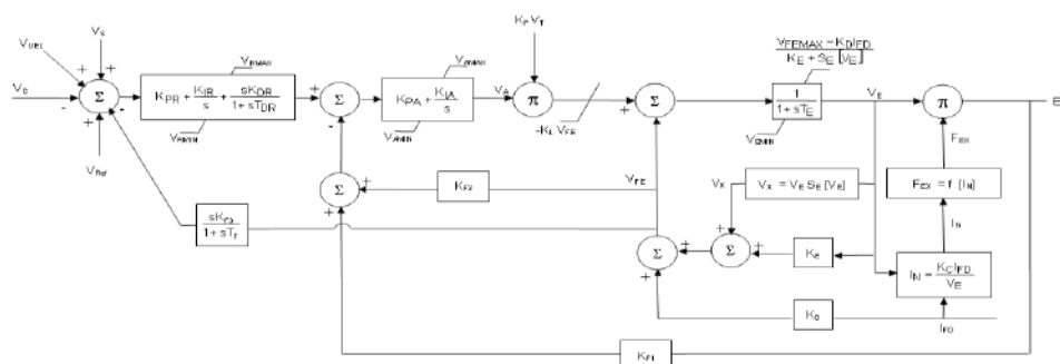
شکل (۳۷-۲): بلوک دیاگرام AVR مدل AC7B
