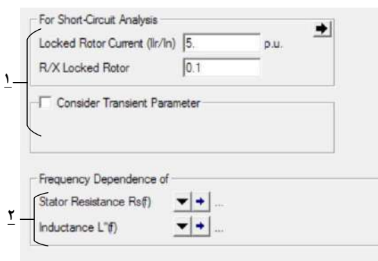
شکل (۶۰-۲): پارامتر مورد نیاز کیفیت توان بخش تایپ مولد DFIG
