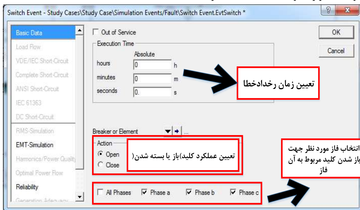
شکل (۵-۱۸): رخداد کلیدزنی
