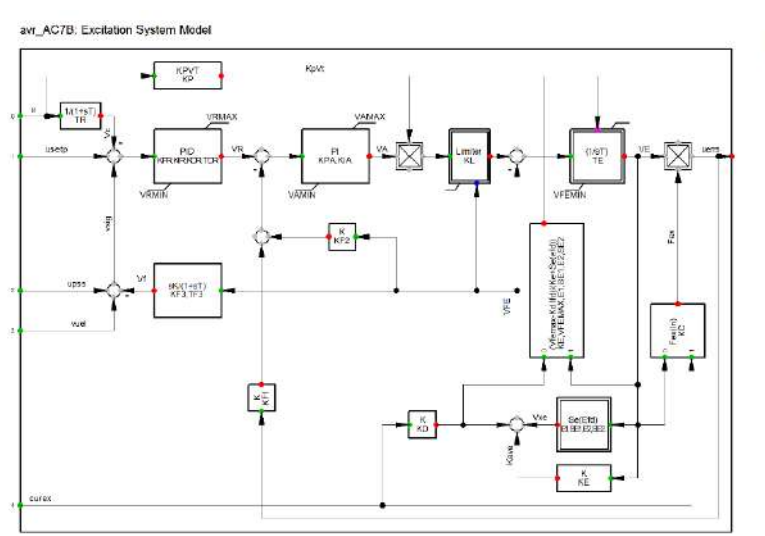
شکل (۲-۳): بلوک دیاگرام AVR AC7B در نرم افزار
