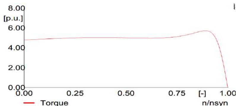
شکل (۵۴-۲): مشخصه گشتاور نسبت به سرعت ژنراتور در مولد DFIG
