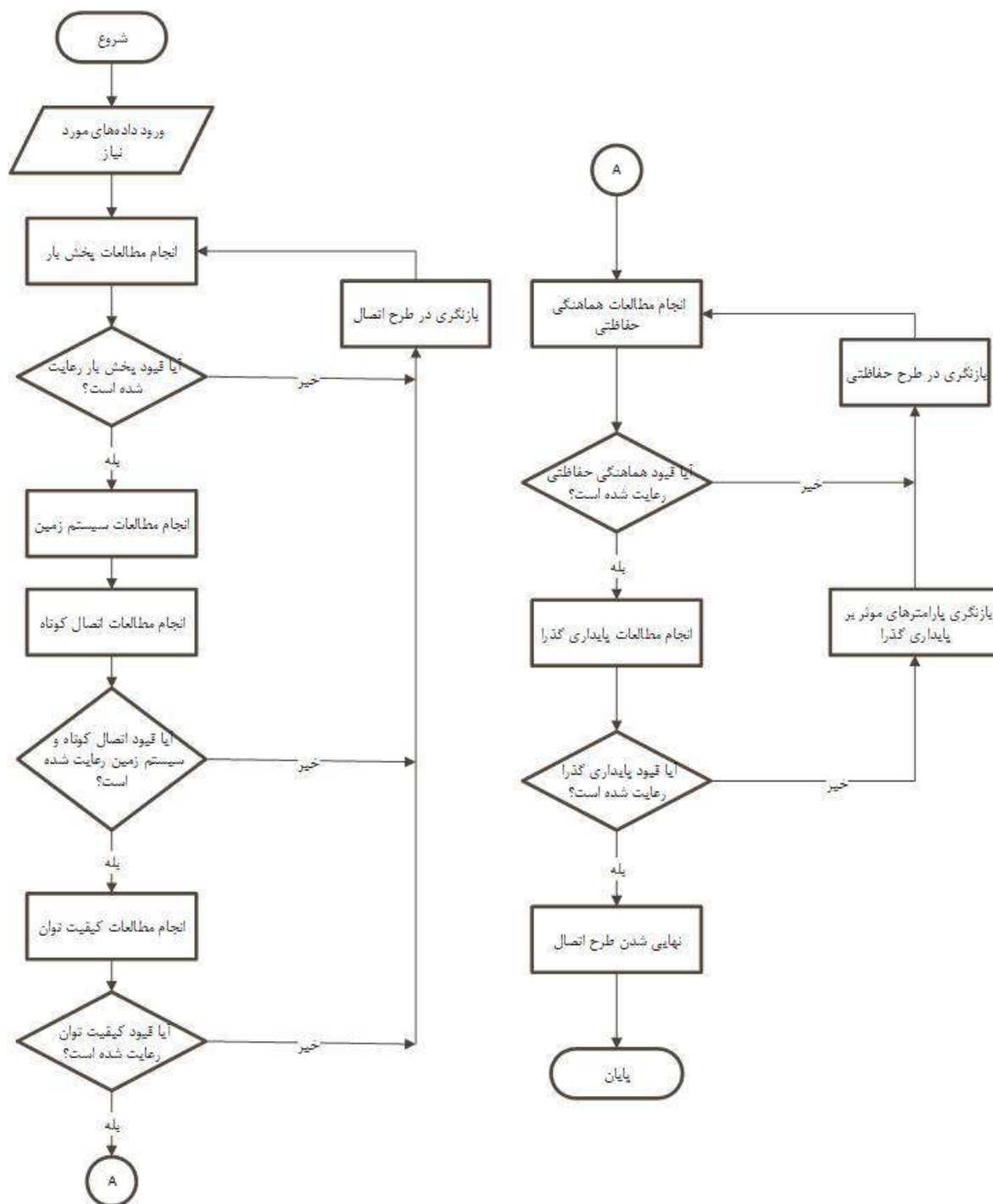
شکل (۹-۱): فلوچارت نحوه انجام مطالعات اتصال به شبکه
