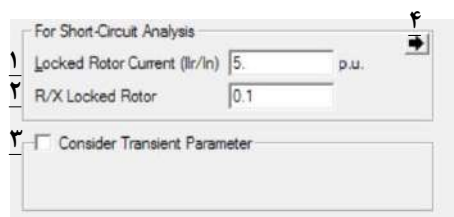
شکل (۵۷-۲): تنظیمات مطالعات اتصال کوتاه بخش تایپ مولد DFIG
