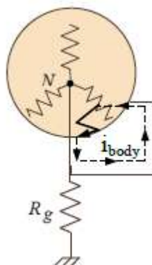
شکل (۸-۲): سیستم زمین TN
