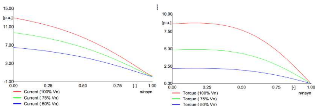
شکل (۵۶-۲): نمودارهای گشتاور و جریان بر حسب سرعت بر واحد مولد DFIG
