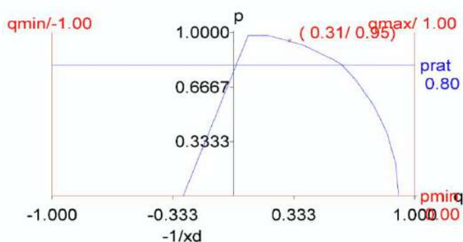
شکل (۷-۲): محدوده مجاز عملکرد ژنراتور سنکرون
