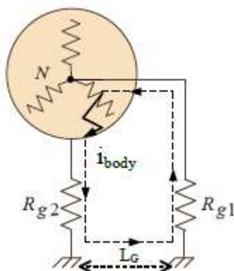
شکل (۸-۱): سیستم زمین TT
