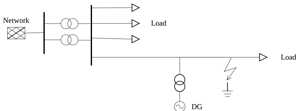
شکل (۴-۸): وقوع خطا در پایین دست مولد پراکنده
