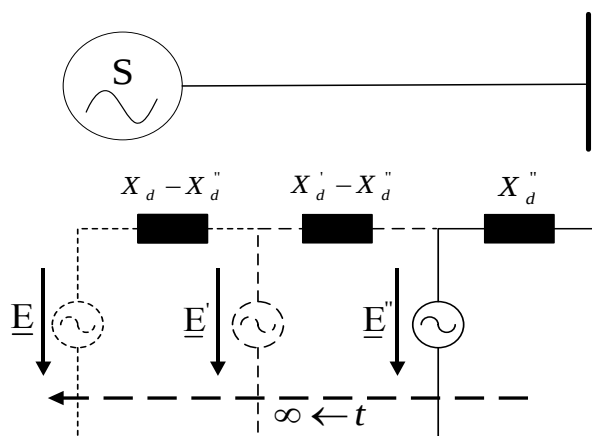
شکل (۲-۱۹): دیگرام مدار معادل تک فاز یک ژنراتور برای محاسبه جریان اتصال کوتاه
