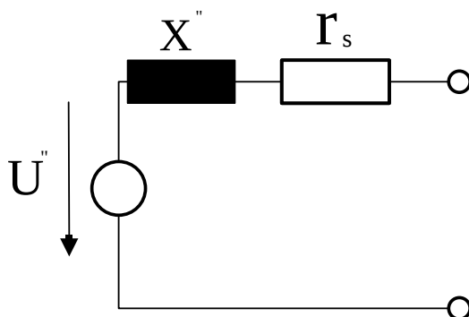
شکل (۴۴-۲): مدل مفهومی مولد DFIG در حالت اتصال کوتاه
