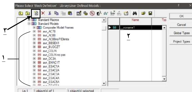
شکل (۳۵-۲): انتخاب یک AVR از پیش طراحی شده برای ژنراتور
