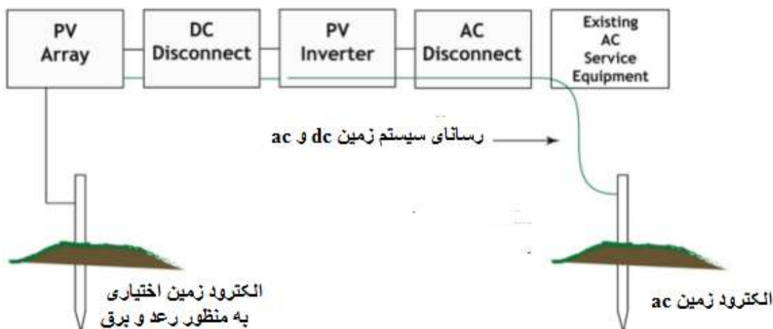
شکل (۸-۴): روش ترکیبی زمین کردن مولدهای فتوولتاییک
