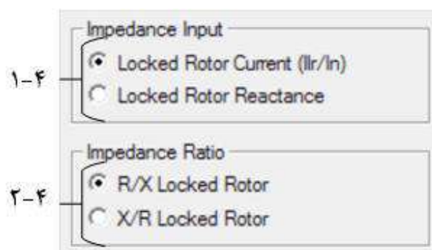
شکل (۵۸-۲): پارامترهای جایگزین مشخصات اتصال کوتاه بخش تایپ مولد DFIG
