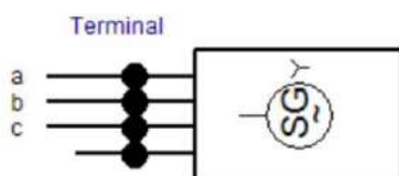
شکل (۵-۲): ماشین سنکرون با رابط خنثی در دسترس
