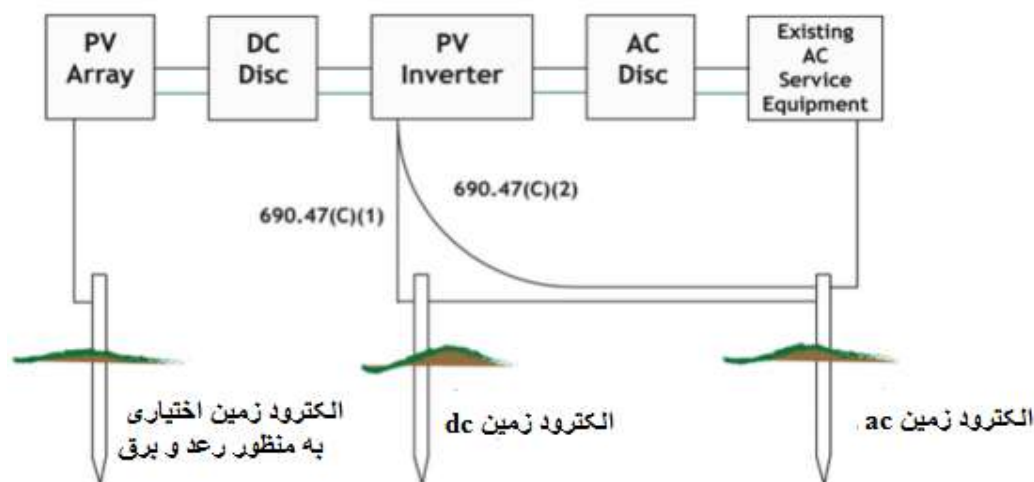
شکل (۸-۳): دو روش زمین کردن مولدهای فتوولتاییک
