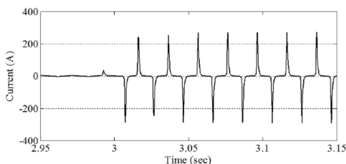
شکل (۴-۶): نمونه شکل موج خروجی ترانس جریان اشباع شده
